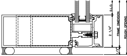
480 JAMB
